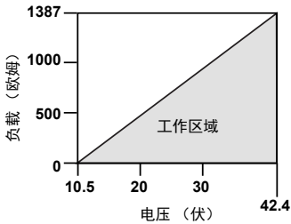
图 5. 回路最大电阻 = 43.5 \times (\text{电源电压} - 10.5)
