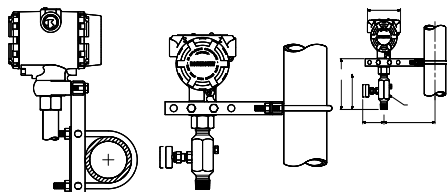
管道安装
