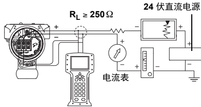
图 3. 工作台连接接线图 (4–20 毫安变送器)
