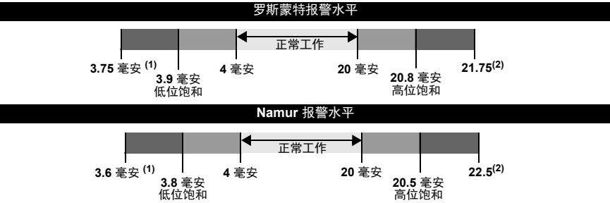
图 6. 报警水平
