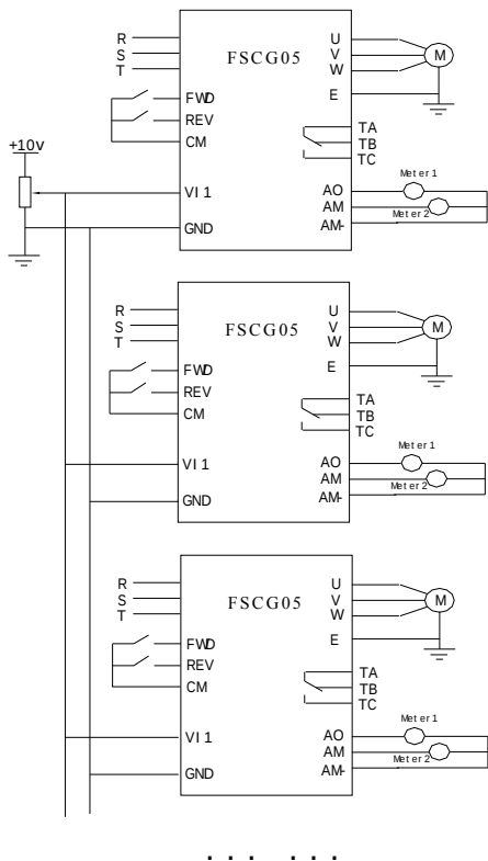
图 7-6 外加电压实现多台变频器的联动运行控制基本接线
