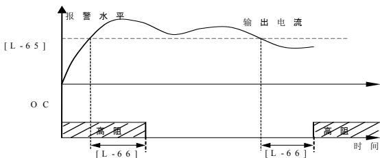
图 5-22 过载报警示意图
