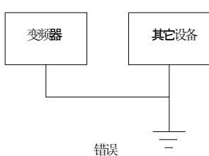
图 2-12 变频器与其它设备接地示意图 3
