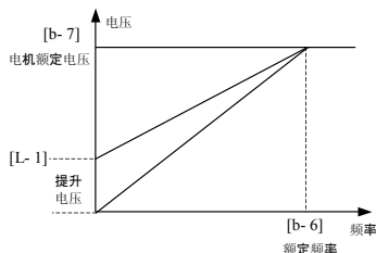
b) 恒转矩曲线转矩提升示意图
