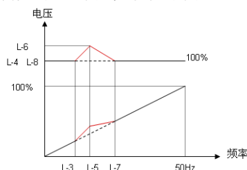
图 5-4 (b) V/F 曲线修正
