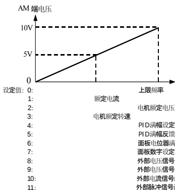
图 5-15 模拟输出端子 AM 的输出内容
