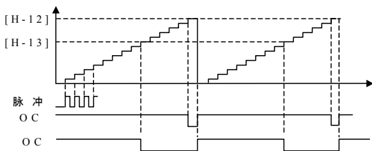
图 5- 27 内部计数器功能
