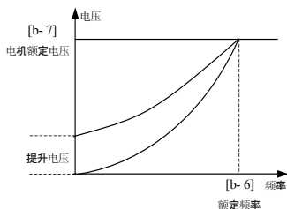
a) 递减转矩曲线转矩提升示意图
