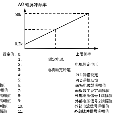
图 5-16 频率输出端子 AO 的输出内容
