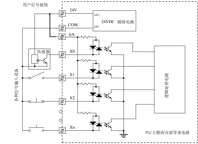
图三 漏型输入接法
