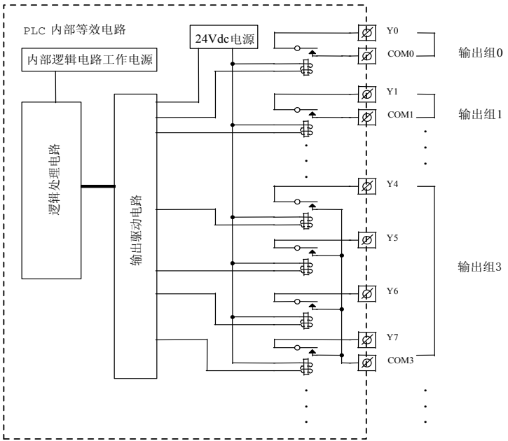
图五 继电器输出等效电路
