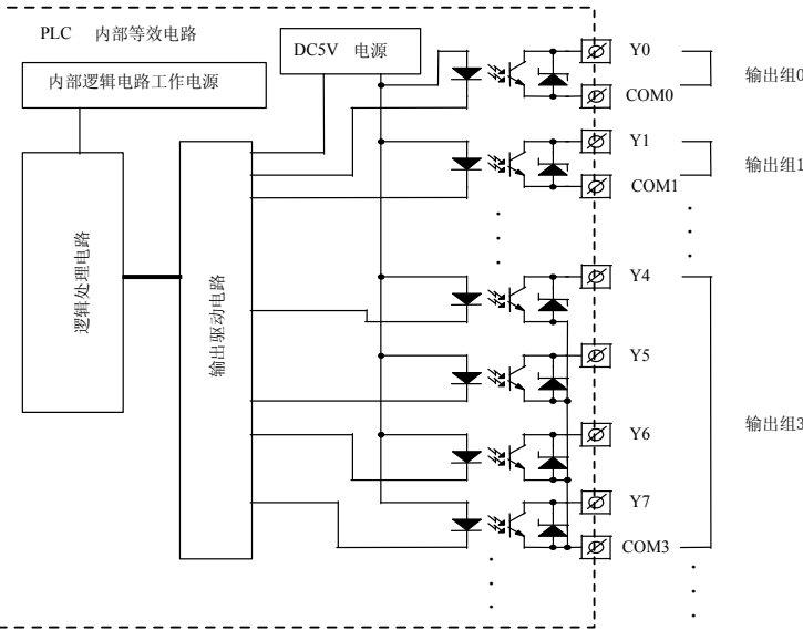
图六 晶体管输出内部等效电路
