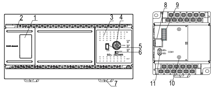
图二 产品构造图
