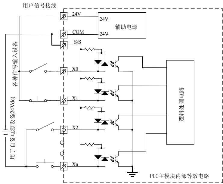
图四 源型输入接法
