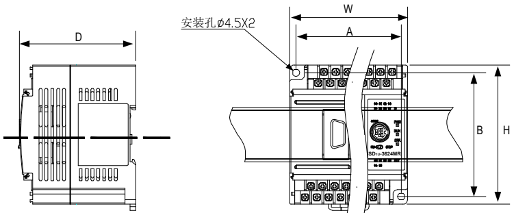
图一 安装尺寸图
