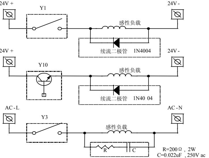
图七 感性负载吸收电路示意图
