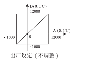
图 3-2 不更改各通道的 D0、D1 值，0 模式对应通道特性
