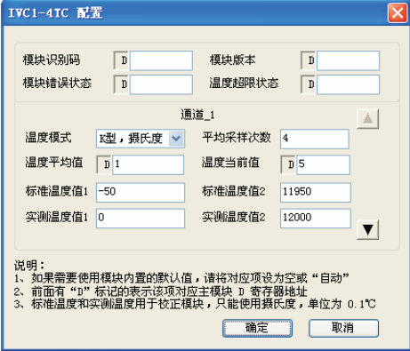
图 4-5 模块第 1 通道设置更改界面
