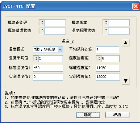
图 4-6 模块第 2 通道设置更改界面
