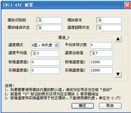
图 4-3 模块第 3 通道设置界面
