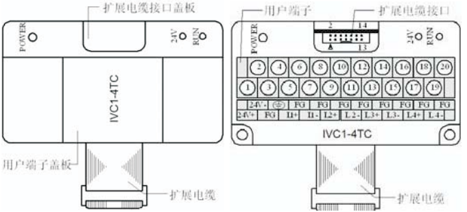
图 1-1 模块接口外观图
