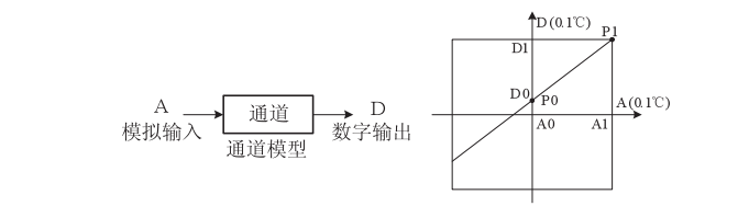
图 3-1 IVC1-4TC 的通道特性示意图
