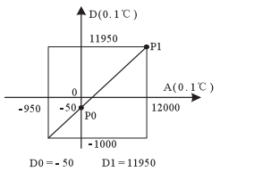
图 3-3 特性更改举例
