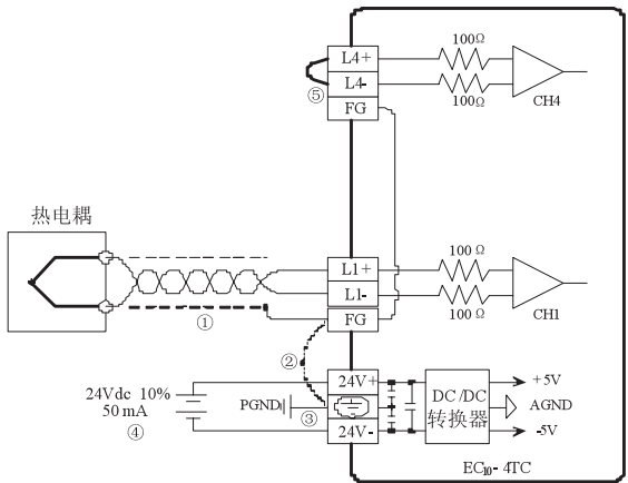
图 1-4 用户端子布线示意图
